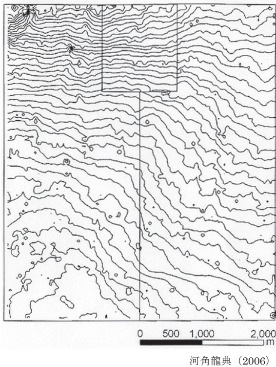
図3 平安時代の平安京城の1m等高線図
