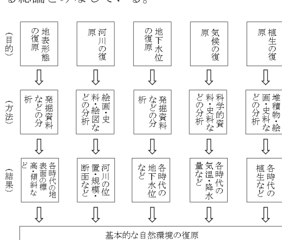
図1 基本的な自然環境復原のフローチャート
